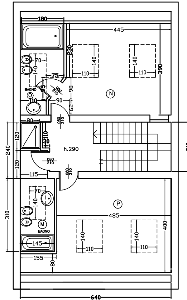
PIANTA PIANO SECONDO
