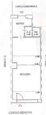
PIANTA PIANO TERRA H. 4,20 m
